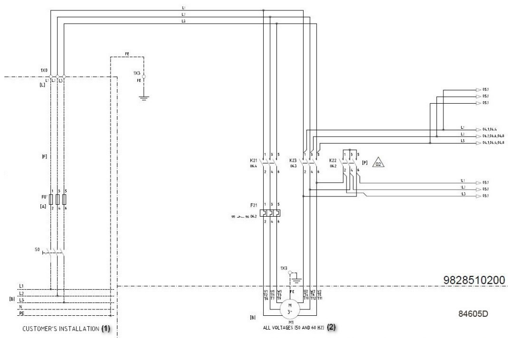
Fig. 13. Conexiunile electrice
