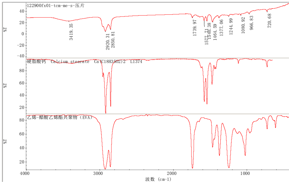
Fig. 1-6 Match FTIR
