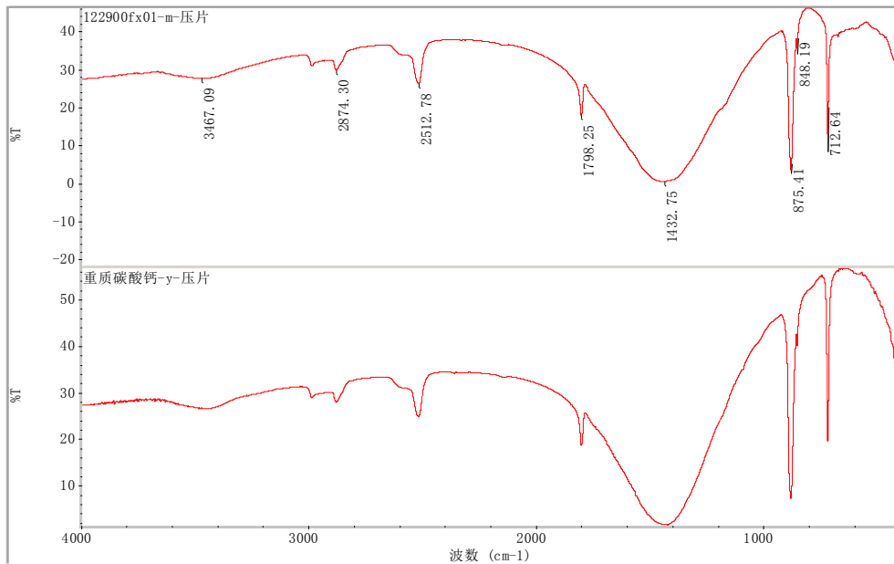
Fig. 1-4 Match FTIR
