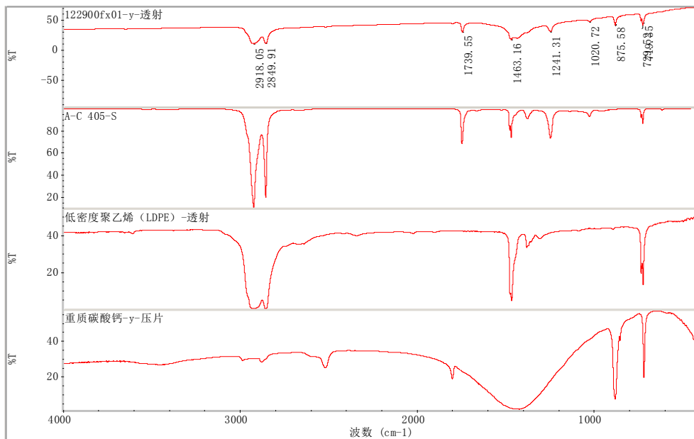
Fig. 1-2 Match FTIR
