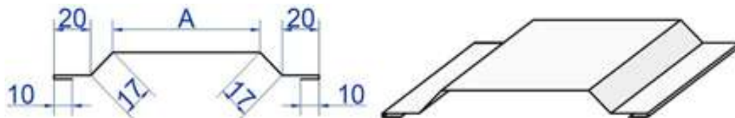
Рисунок 40. Фигурный нащельник
