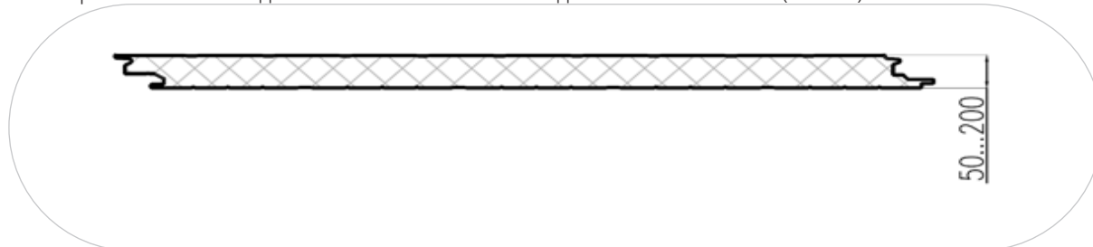
Рисунок 19. Геометрия стеновой сэндвич-панели с замковым соединением SECRET FIX (ПСТ SF).
