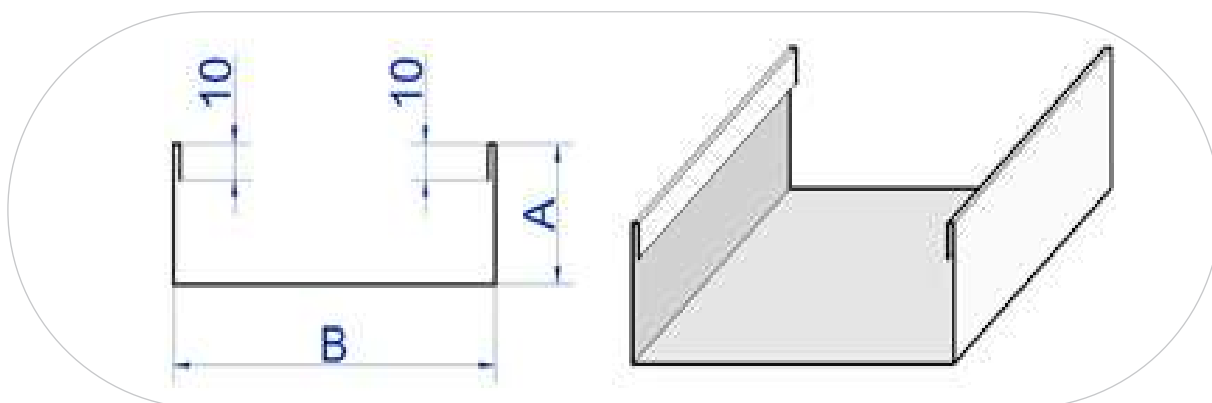
Рисунок 36. Направляющая (швеллер) для панелей
