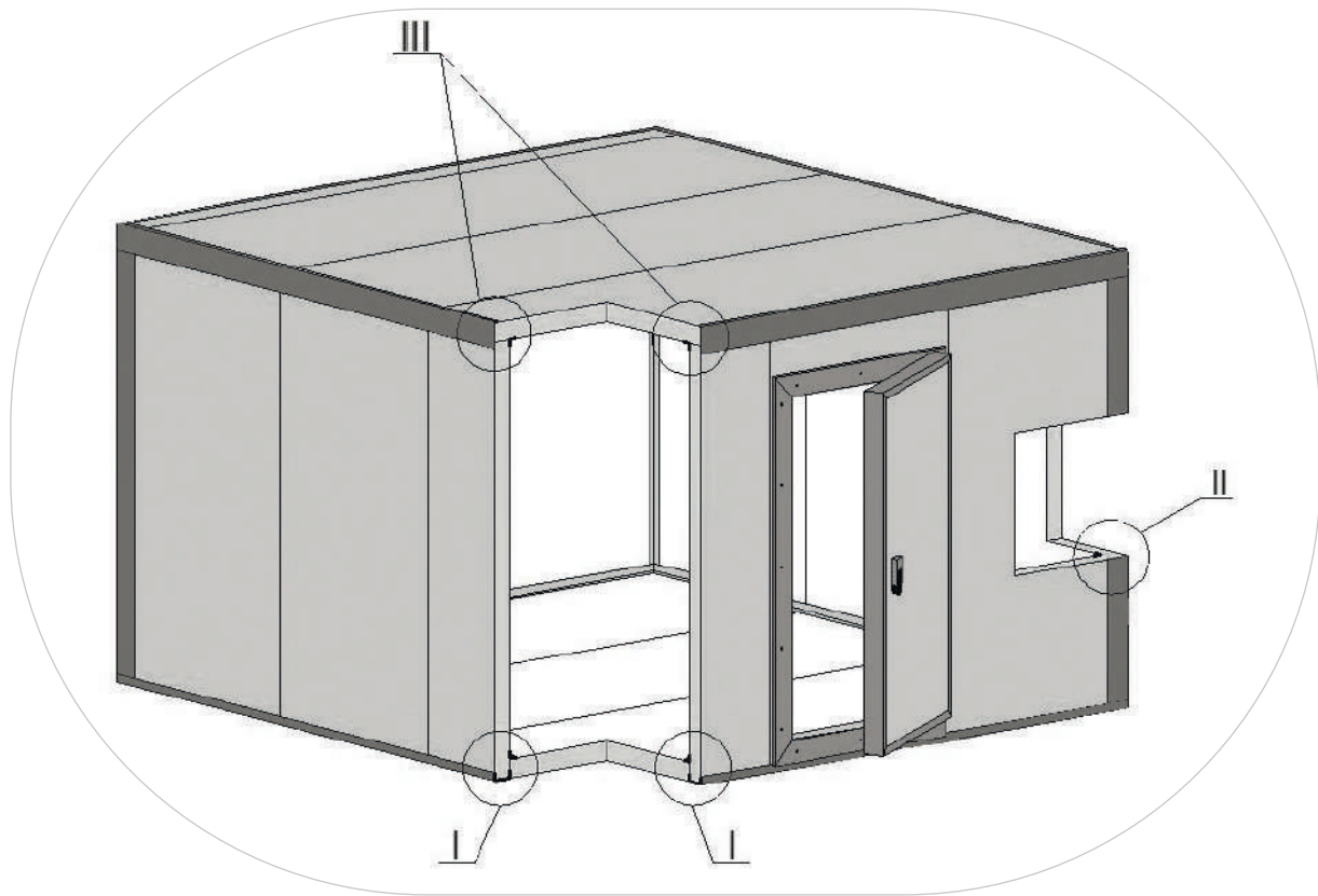
Рисунок 30. Схематическое изображение холодильной камеры I. узел стыковки панелей для пола и стеновых сэндвич-панелей II. узел стыковки стеновых панелей III. узел стыковки потолочных и стеновых панелей
