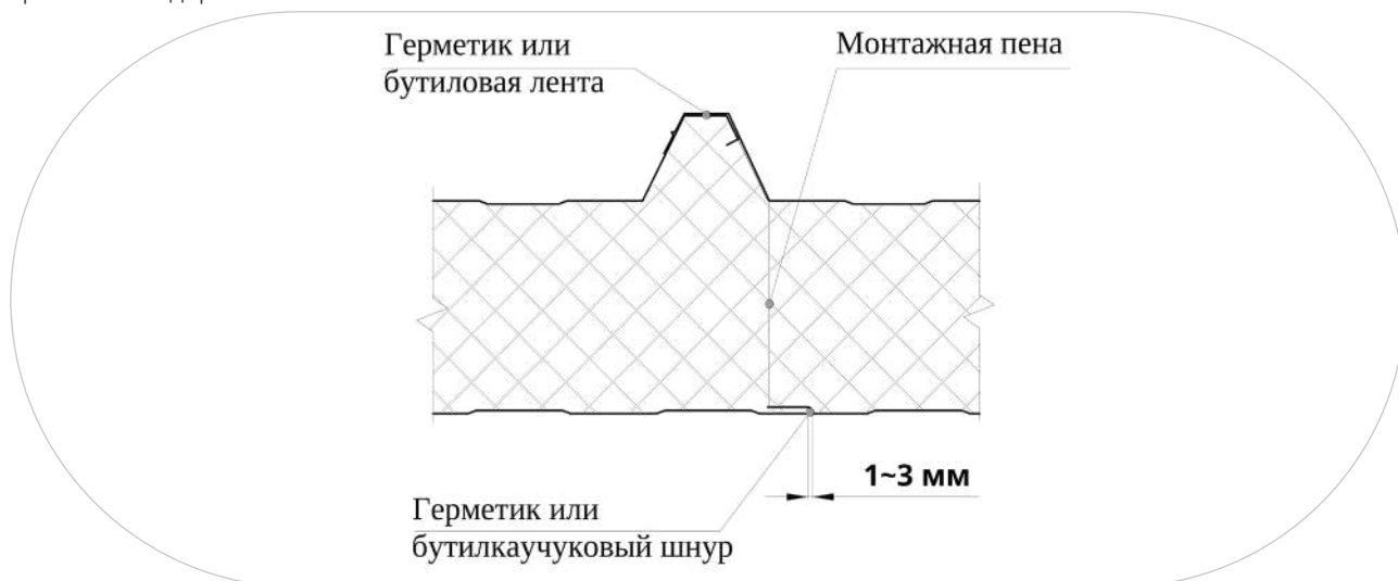
Рисунок 22. Стык кровельных панелей со стандартным замковым соединением. Для обеспечения лучшего прилегания панелей к прогонам в местах соединений панелей рекомендуется производить крепление саморезов через кровельный держатель.
