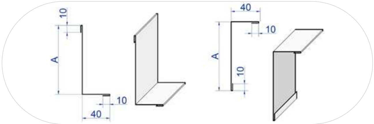
Рисунок 39. Уголки неравносторонние (для стыков потолочных и стеновых панелей)
