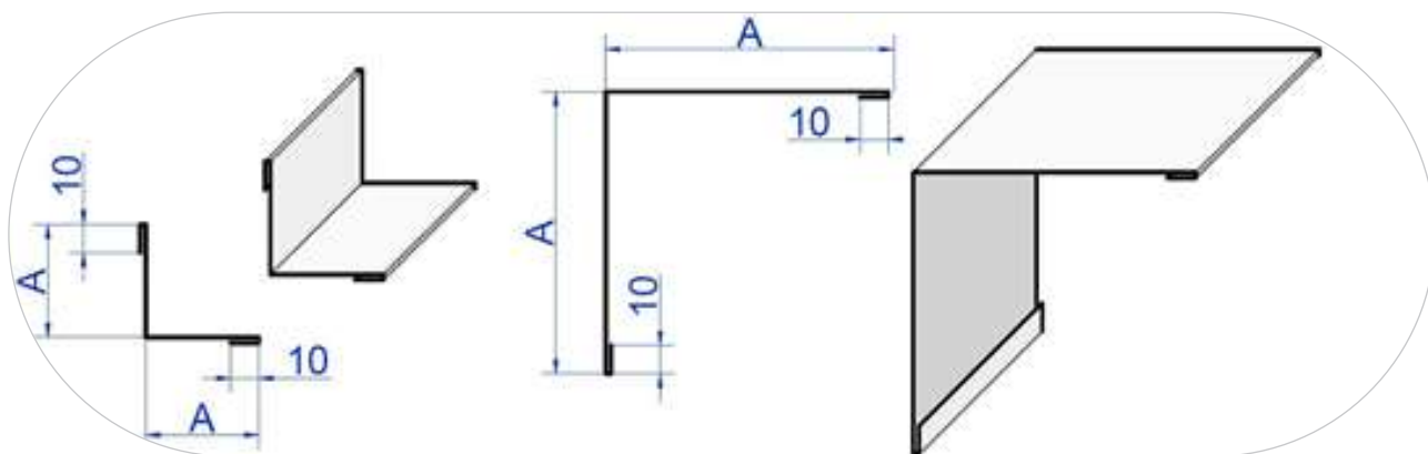
Рисунок 37. Равносторонние уголки (плоские)
