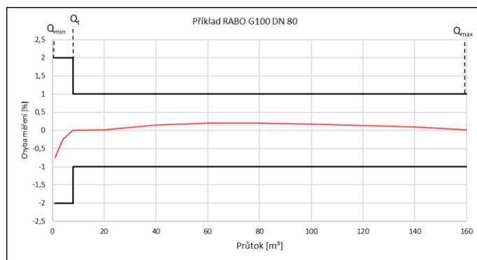
Obr. 13 | Meze chyb
