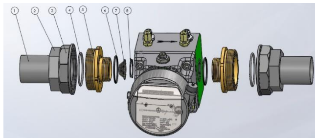
Рис. 8 | Соединительные детали для типа RABO-СТ
