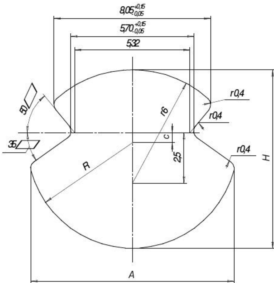
Рисунок 1 - Размеры фасонного провода
