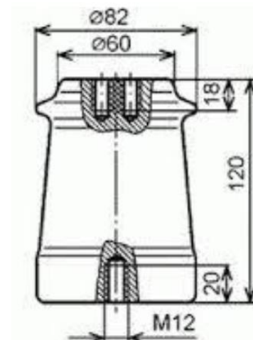
Изолятор ИО-10
