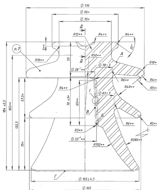
Изолятор ШФ-20ГО (ШФ-20-13-2-I)
