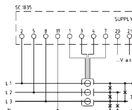
Q52D3L063X4C2 - Q52D3L125X4C2 system 3 fazowy, 4 przewodowy for three-phase four wires system
