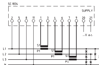
Q52P3L005X4C2 system 3 fazowy, 4 przewodowy for three-phase four wires system
