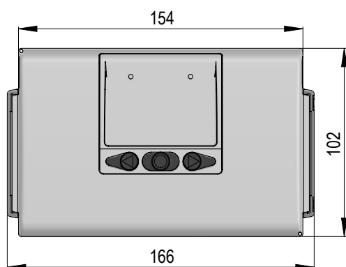
Dimensiunile calculatorului MULTICAL® 603
