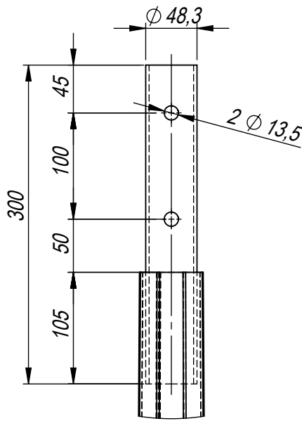
DETAY X ÖLÇEK: 1/5
