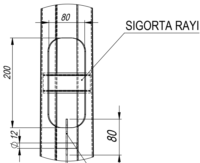
DETAY B ÖLÇEK: 1/5
