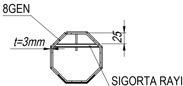
KESİT A-A ÖLÇEK: 1/5
