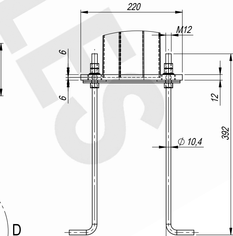
DETAY D ÖLÇEK: 1/5
