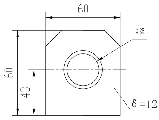
Позиция 7 - Кольцо для подъема крышки
