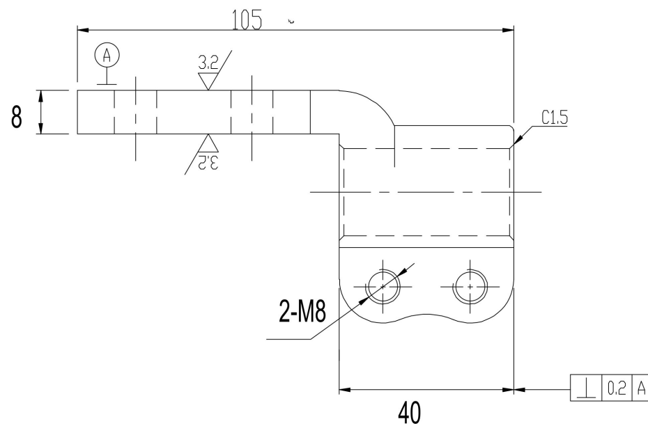
Позиция 4, 5 - Клемма
