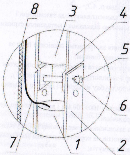
Малюнок 6. З'єднання блоків анодного заземлювача в гірлянди.
