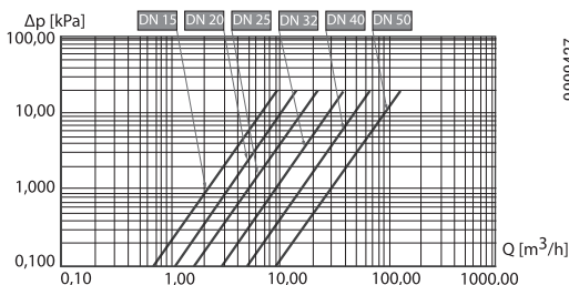
Charakterystyki parametrów pracy zaworów ONYX PN40
