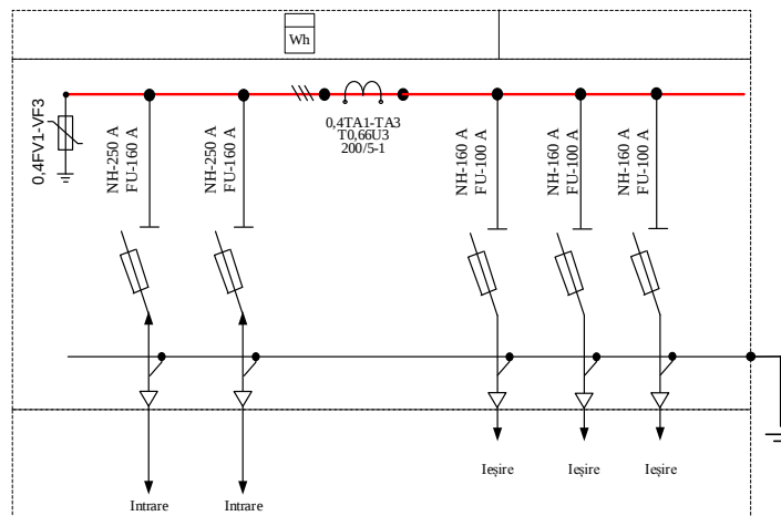
nr. 3. Schema monofilară a PPDÎTV cu 5 aparate de comutație
