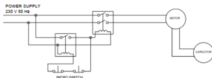
Рис./Fig №4. Электрическая схема
