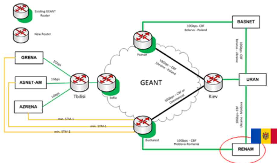
Fig. 2. Schema arhitecturii rețelei regionale propusă în proiectul „EaPConnect
