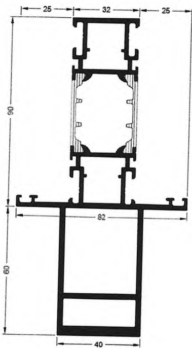
491 500 Profilé structure 32/82
