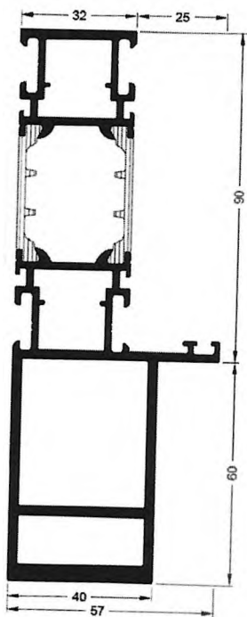
491 660 Profilé structure 32/57
