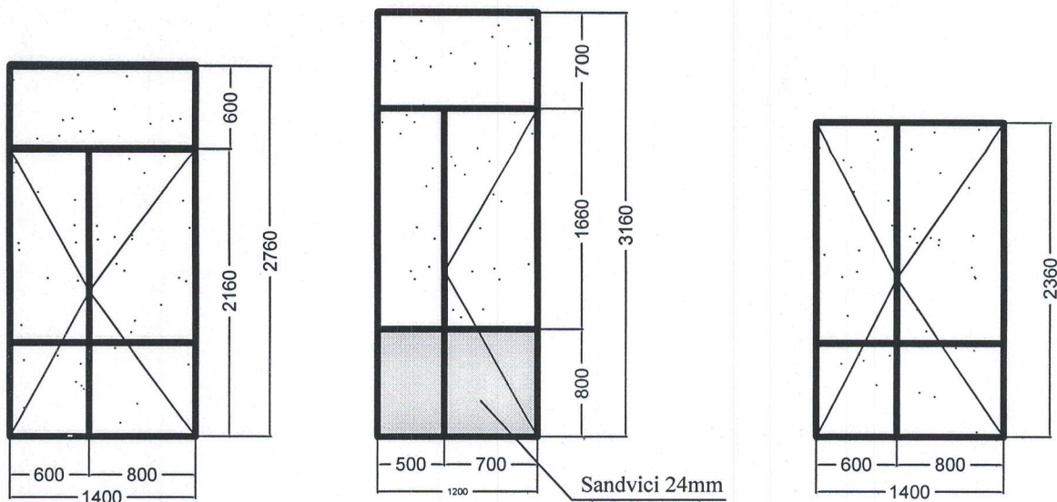
Usa Auditorii-10buc
