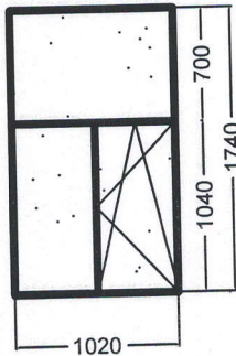
Ferestre 2 buc
