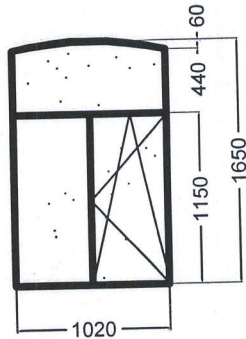
Ferestre 25 buc
