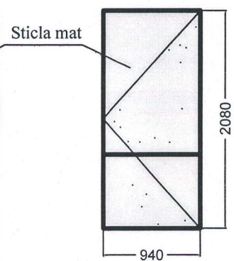
Usa auditorii-1buc
