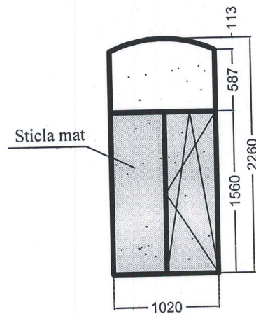
Ferestre 5 buc
