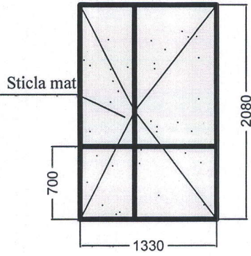
Usa auditorii-2buc
