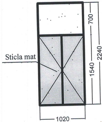
Ferestre 2 buc
