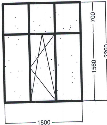
Ferestre 8 buc
