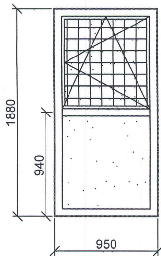
Ferestre; 950-x1880(h) -1buc
