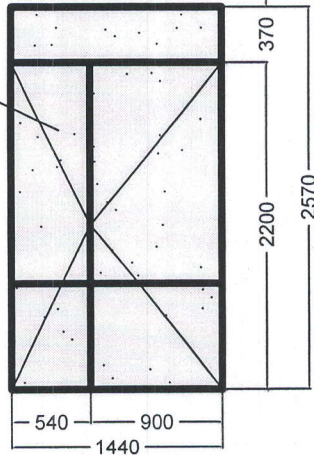
Usa auditorii-1buc
