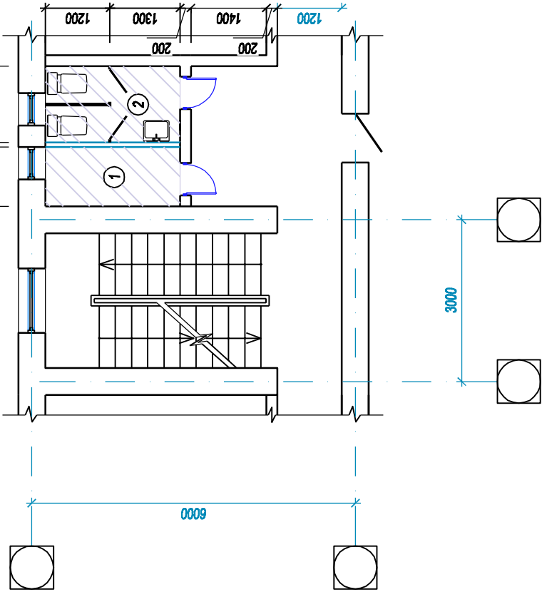
Plan finisare a tavanului etaj I ; III
