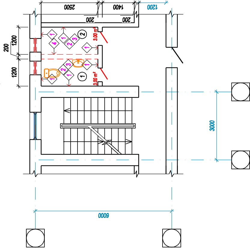
Plan etaj III
