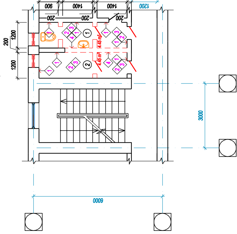
Plan etaj II
