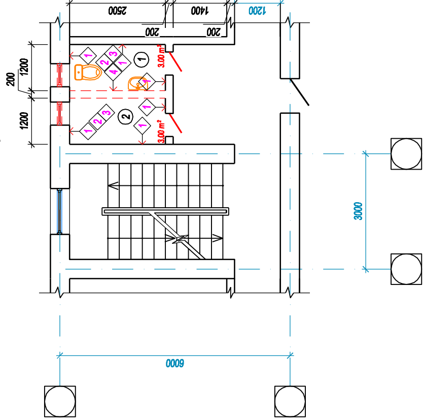
Plan etaj I
