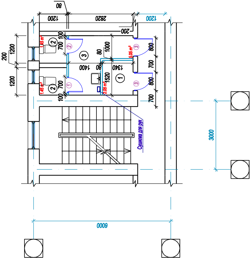
Plan soclu; etaj II
