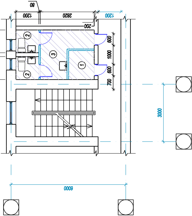
Plan finisare a tavanului soclu; etaj II
