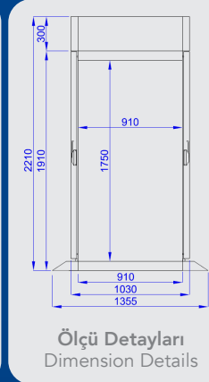
Ölçü Detayları Dimension Details
