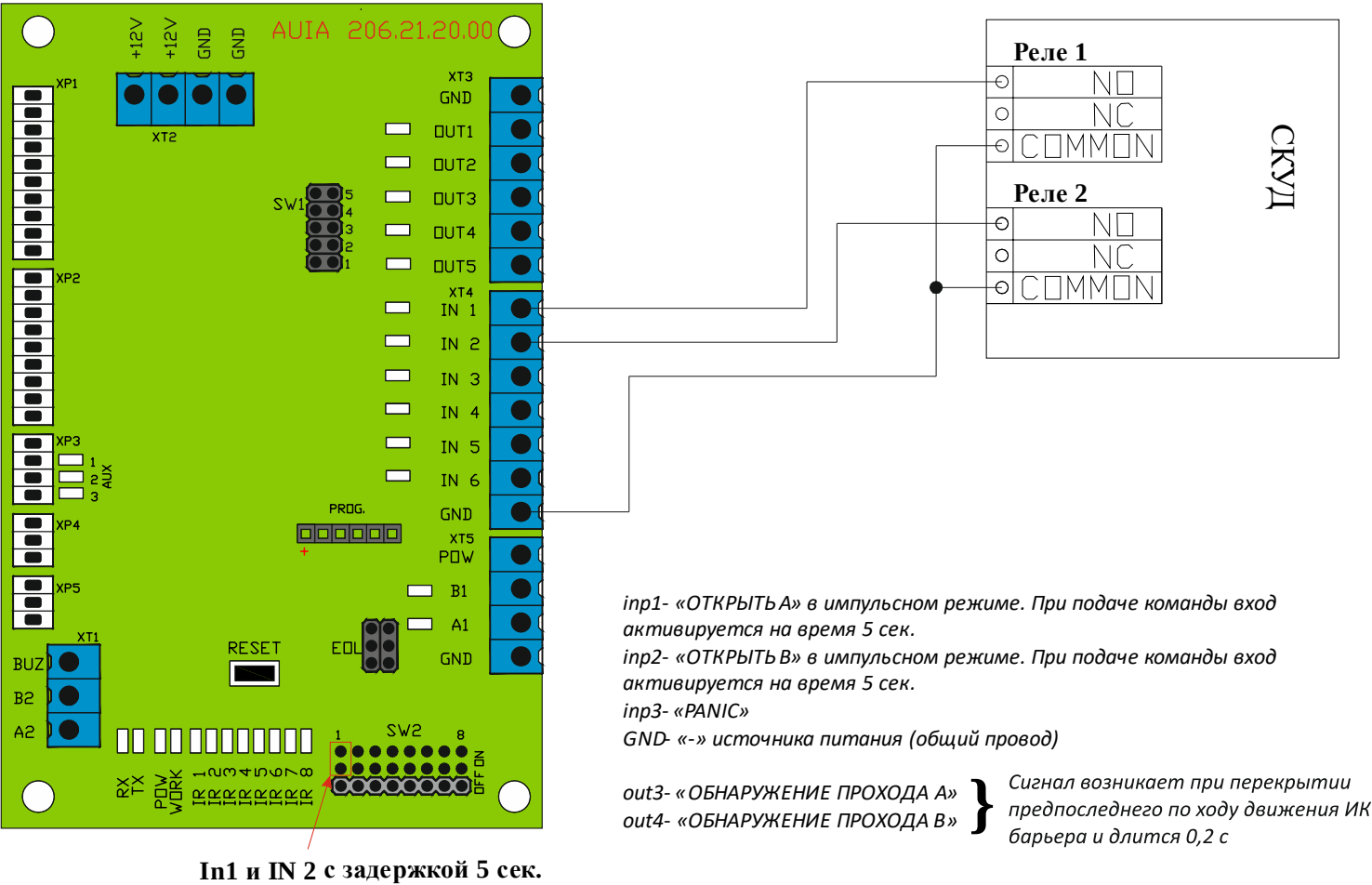
Схема электрическая подключения турникета к системе контроля и управления доступом (СКУД)
