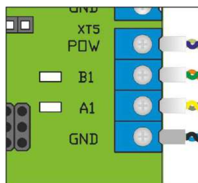
Рис.18– Подключение кабеля связи с пультом управления к клеммам РСВ.206.21.00.00
