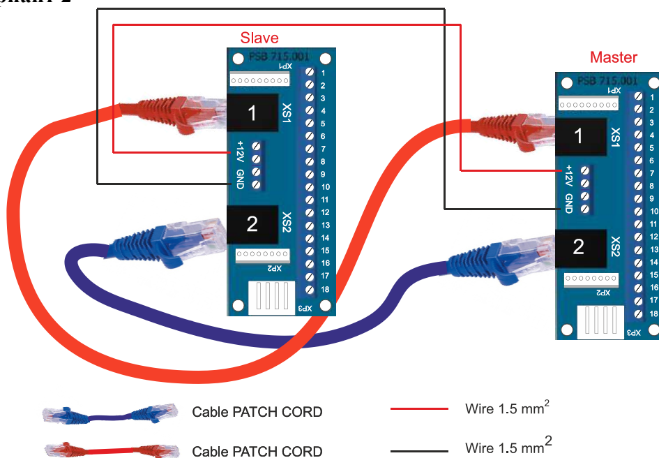
Рис. 15 – Варианты подключения кабелей между тумбами Master и Slave турникета «Speedblade-1»
