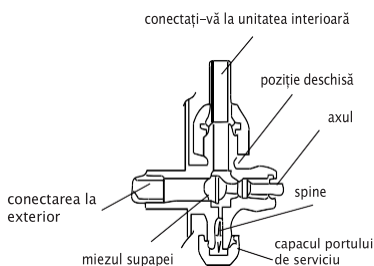
Diagrama supapei cu 3 căi
