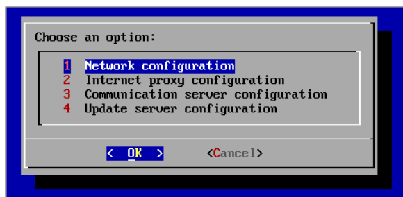
Interfața de configurare Security Server (meniu principal)
