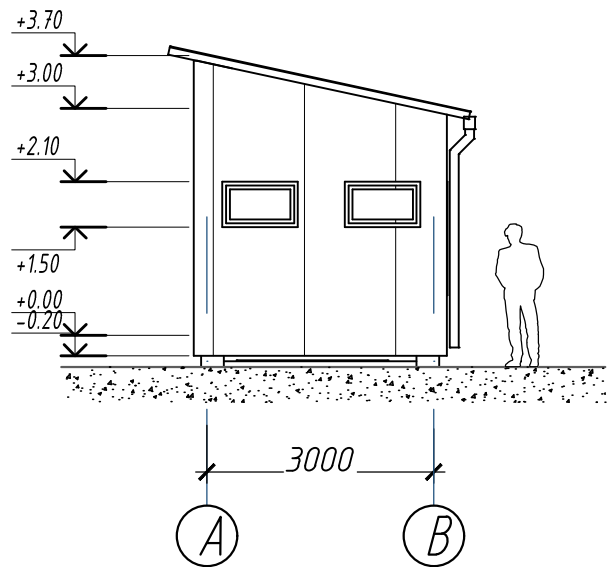
Fatada A-B
