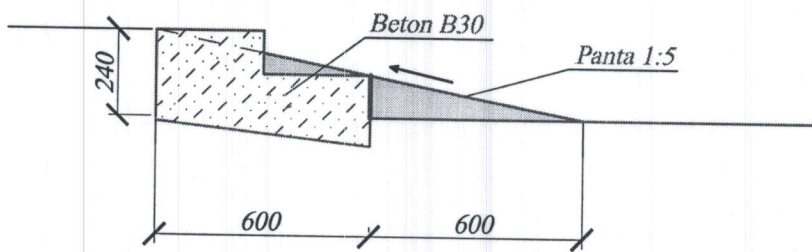
Sectiune II - II
