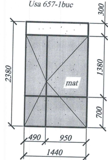
Usa 648-1buc
