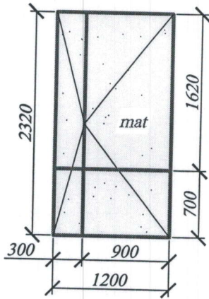
Usa 628-1buc
