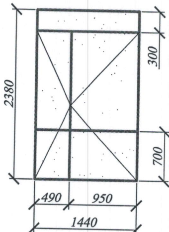
Usi 644,645,646,647-4buc
