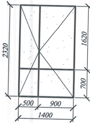
Usa liceu Et.1-1buc
