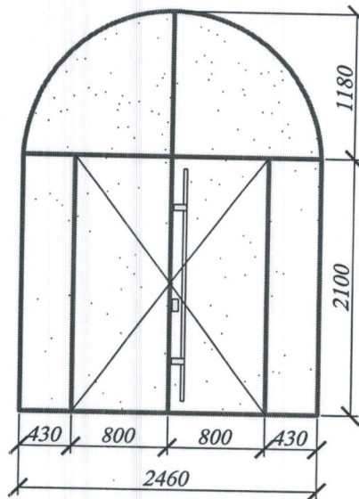
Glasvandri cu usa-1buc
