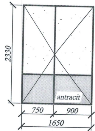
Usa demisol -1buc
