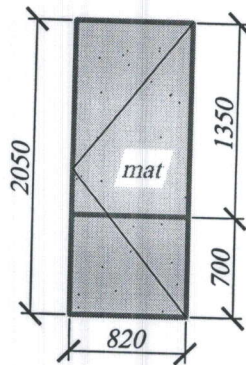
Usi 657-1buc
