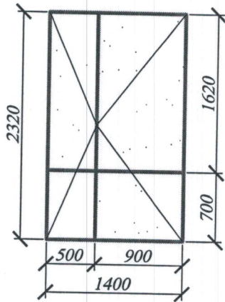
Usi 625,626,627,628-4buc
