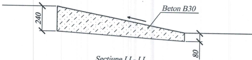
Sectiune II - II
