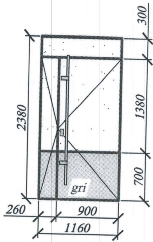
Usa intrare Luceu-1buc
