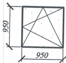
Ferestre -4buc
