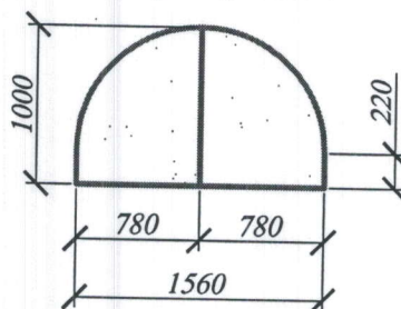
Fereastră-1buc
