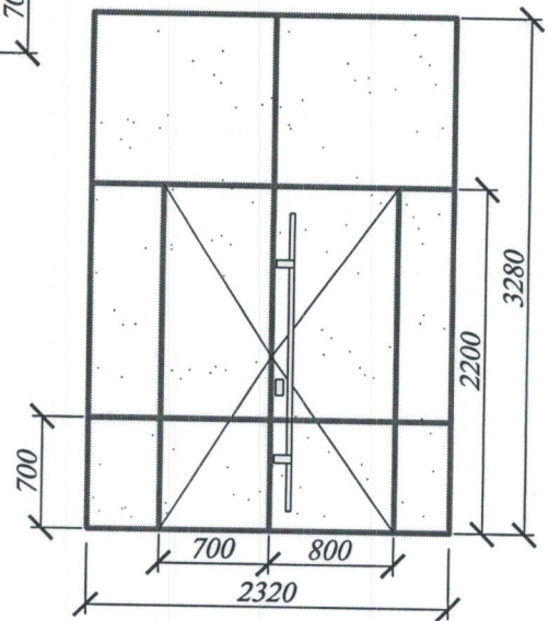
Glasvandri cu usa-1buc
