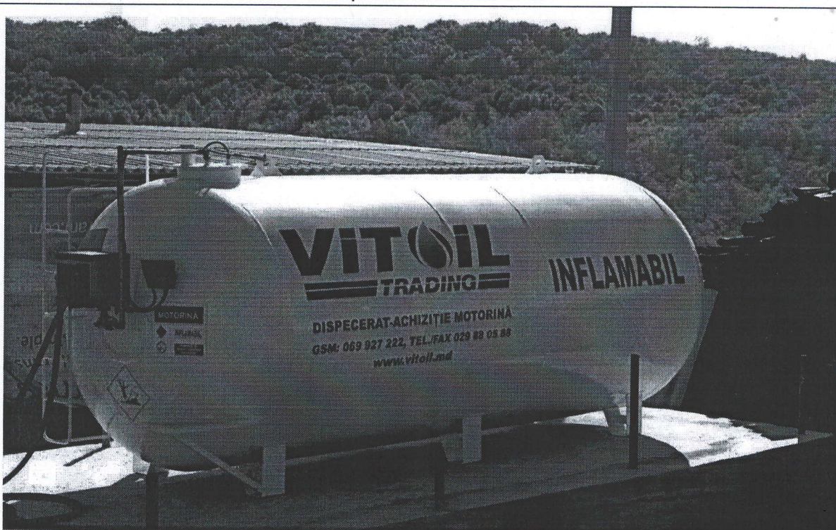
Statie pe baza rezervorului 16 mc
