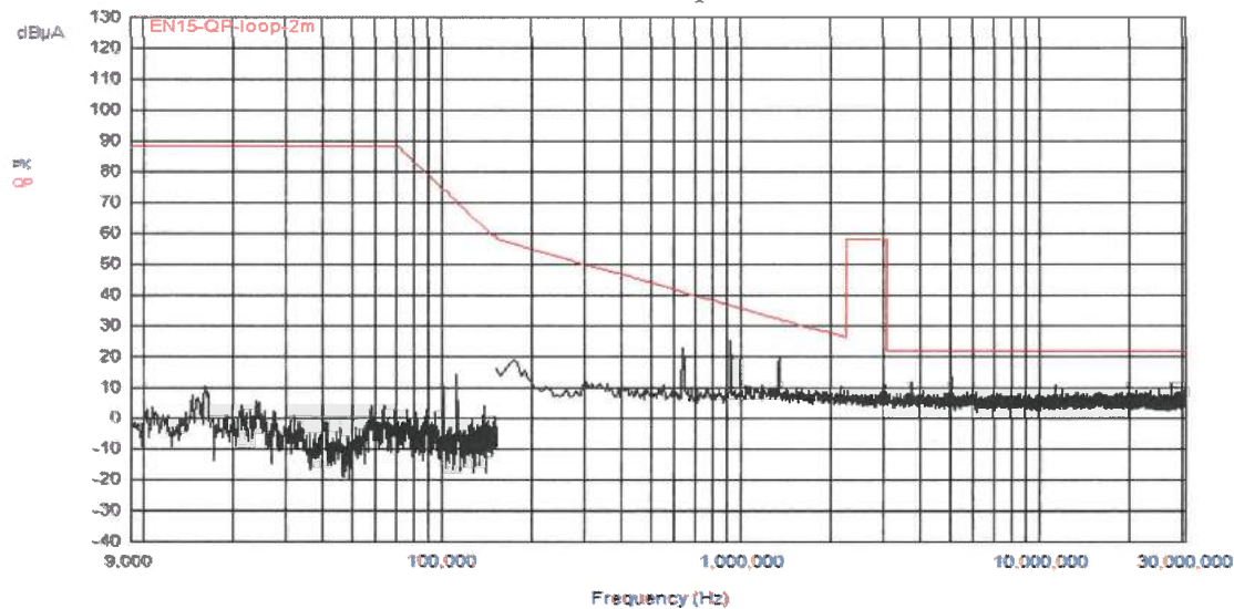
Perturbatii radiate pe axa Z
