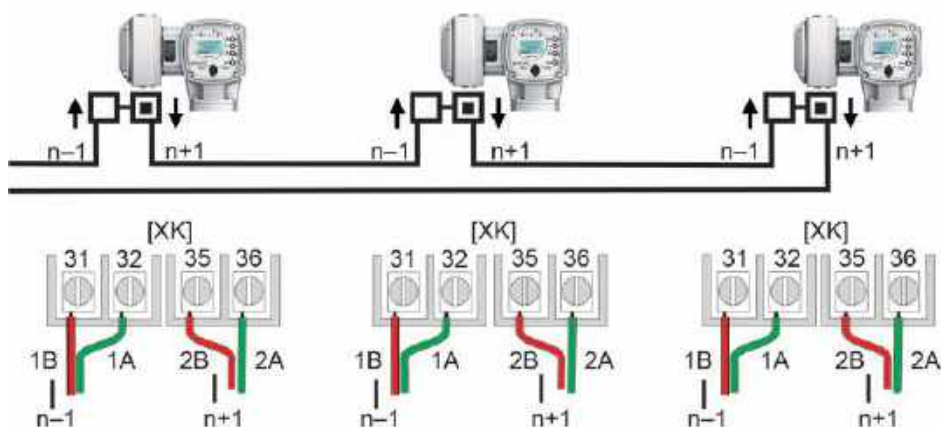
Imagine 39: Alocarea bornelor la topologia tip inel (cu 2 canale):
