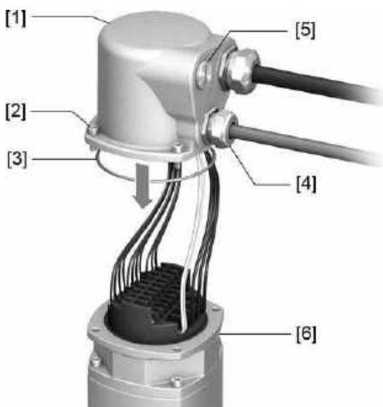
Figura 18: Închideți compartimentul terminal
