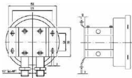
Local, montare pe perete Montare locală pe perete
