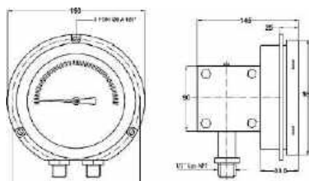
Montare pe panou prin intermediul unei flanșe frontale cu 3 orificii Montare pe panou printr-o flanșă frontală cu 3 găuri
