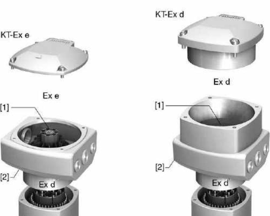
Figura 24: Conexiune electrică KT / KM
