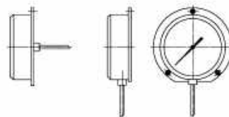
A parete, ancorato a mezzo di una flangia a 3 fori posteriore Panel mounting, through a 3 holes rear flange
