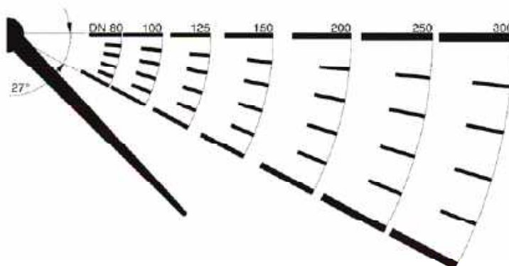
27° = 1/10 dell'estensione angolare della scala 27° = 1/10 of angular scale extension
