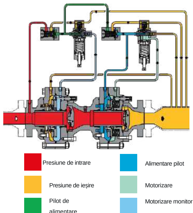
Figura 6 ASX 176/FO cu PM/176
