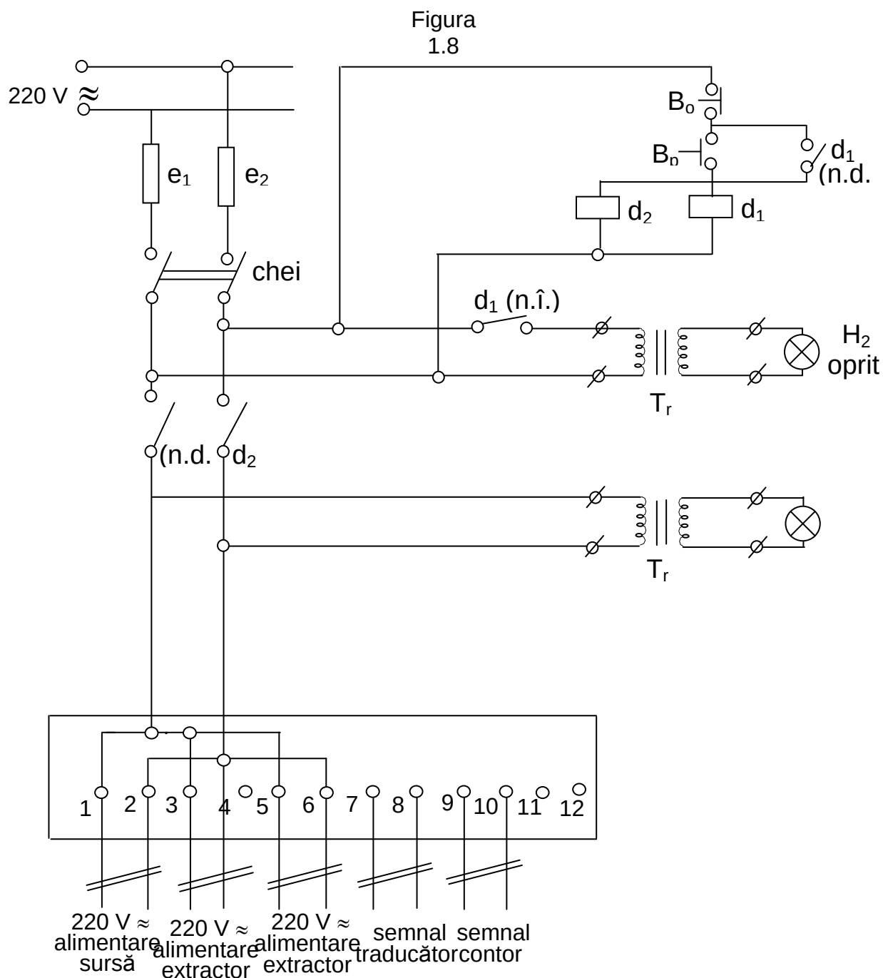
Fig. 10. Schema electrică de acționare pentru măsurarea debitelor gazelor: e1, e2 - siguranțe; H1, H2 - lămpi de semnalizare; B - buton pornire; B0 buton oprire; Tr - transformatoare; d1d2 - bobine contactoare.
