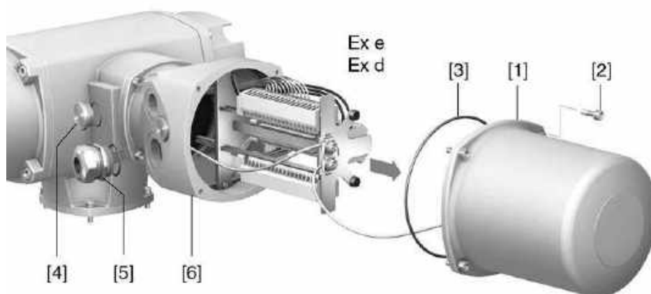
Imagine 27: Deschiderea compartimentului de conectare
