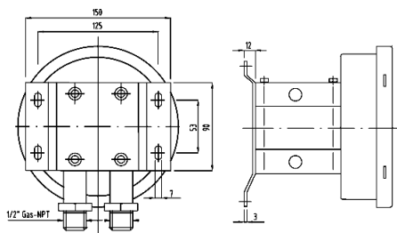
Montaggio locale, a parete Local wall mounting
