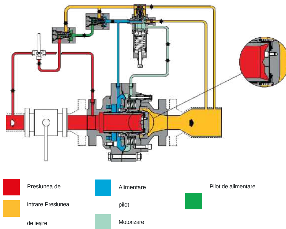
Figura 7 ASX 176/FO cu amortizor de zgomot LDB/176
