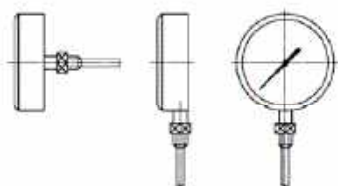
Montaggio locale, diretto su tubazione Local mounting directly on pipe
