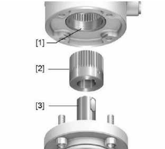
Proiecta Figura 9: Fixarea supapei prin cuplaj
