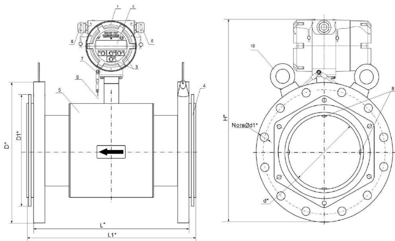
Рис.16. Вид расходомера DN25-DN300 (ППР фланцеванный, с защитными кольцами).
