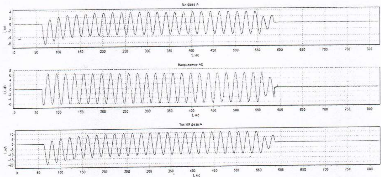
Рис. 9.2 Осциллограмма № 137984
