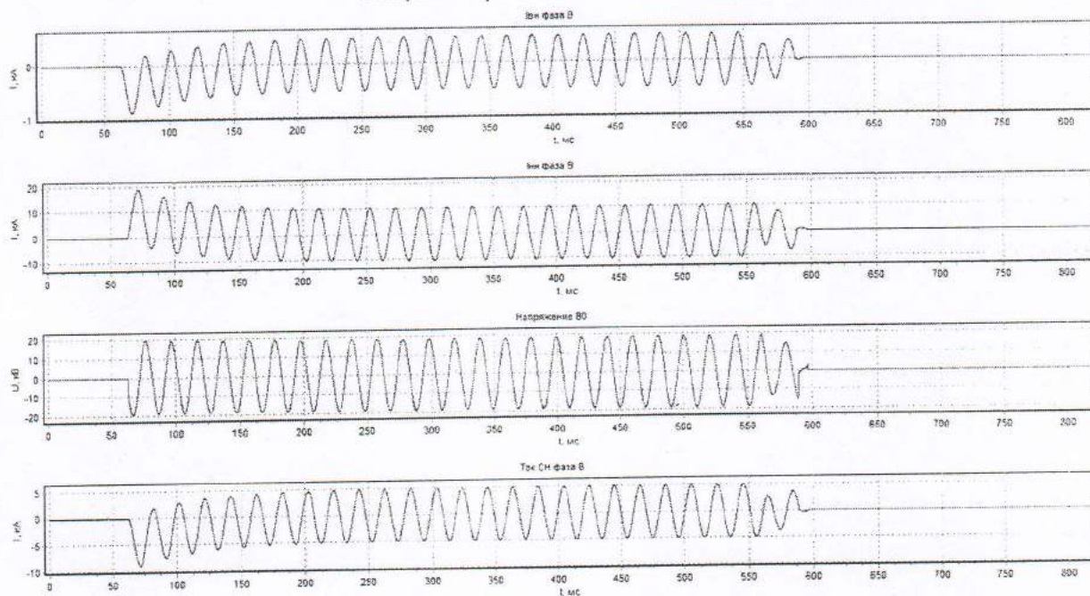
Осциллограмма № 138000
