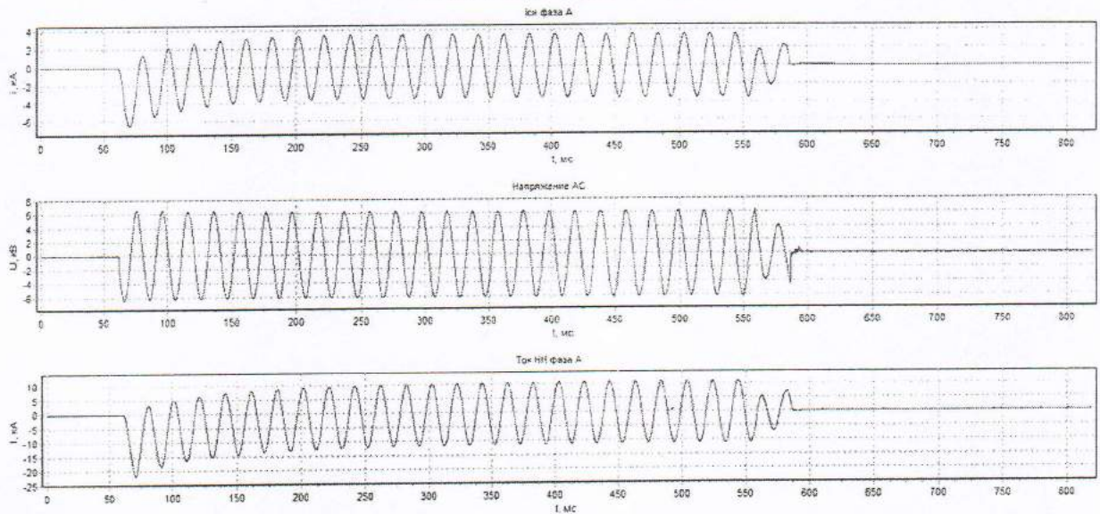
Рис. 9.1 Осциллограмма № 137983
