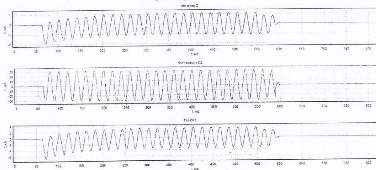
Осциллограмма № 137992
