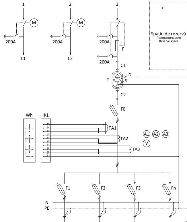
Рис. 1 Схема GALBOX
