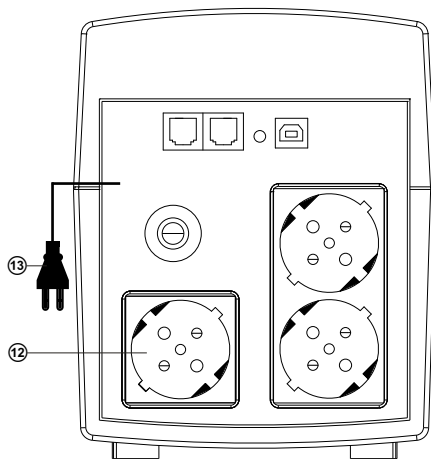
Задня панель ДЖБ Pro 1000 (USB)/Pro1500 (LCD, USB)
