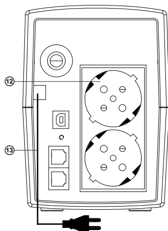
Задня панель ДЖБ Pro 600/800/650 (LCD, USB)
