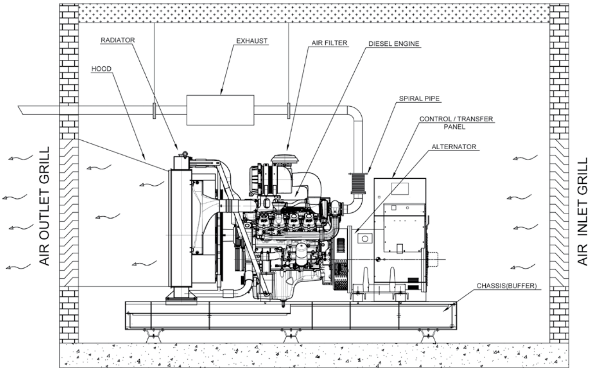
УСТАНОВКА ГЕНЕРАТОРА - БЕЗ КАБИНЫ ПЛАН РАЗМЕЩЕНИЯ 1
