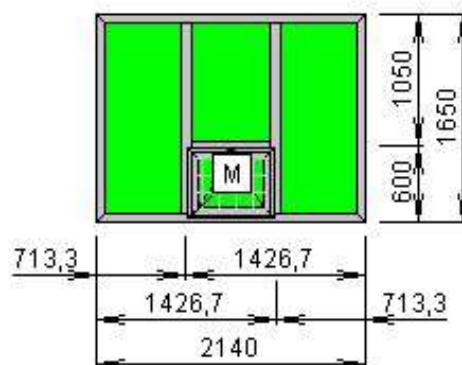
Изд. №4 Кол-во 2 шт.
