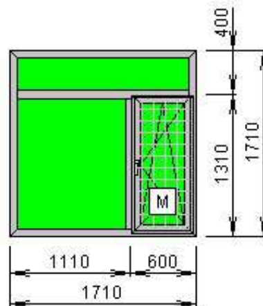
Изд. №2 Кол-во 1 шт.
