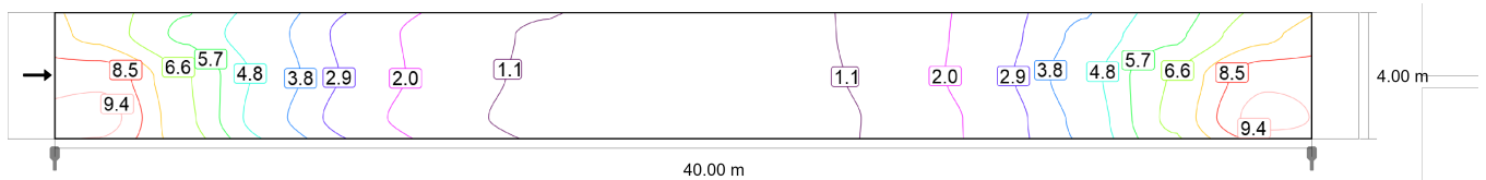
Valoarea de întreținere, intensitatea de iluminare orizontală [lx] (Linii Isolux)
