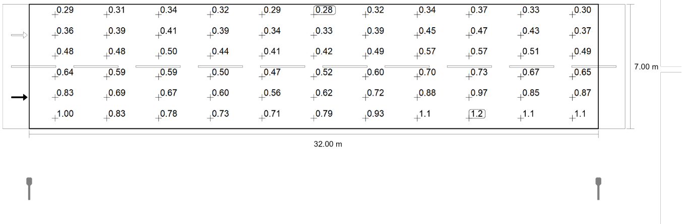
Observator 1: Densitatea luminii la instalația nouă [cd/m 2 ] (Raster valoric)
