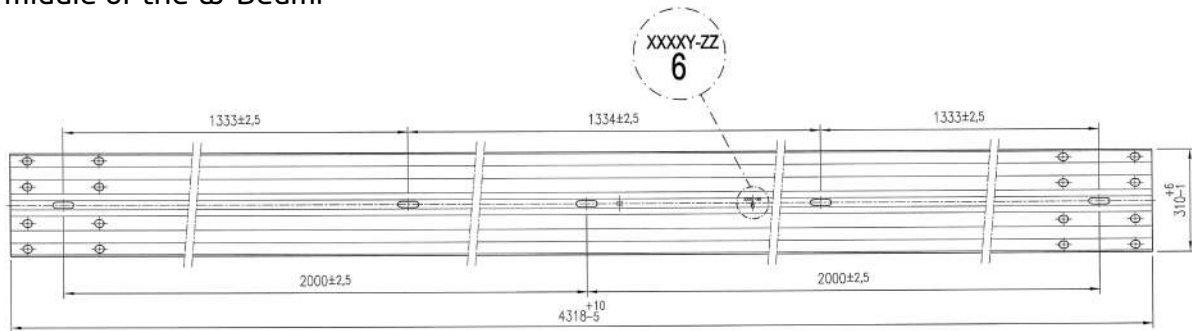
W-Beam
