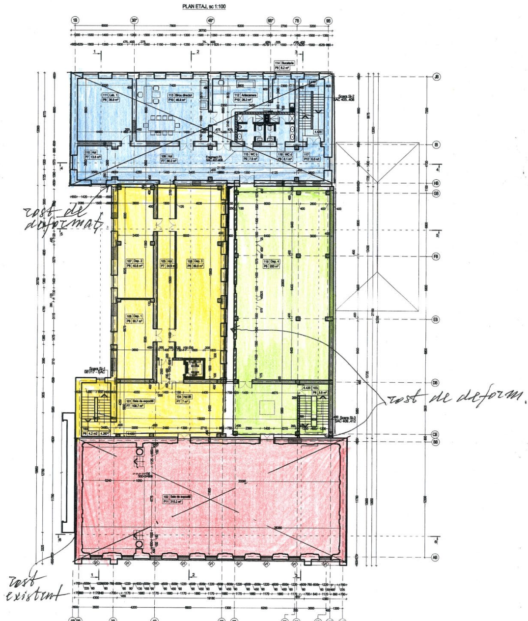
fig. 12 Plan etaj. Schema dispozitiei cladirii la blocuri seismice cu rosturi de deformatie
