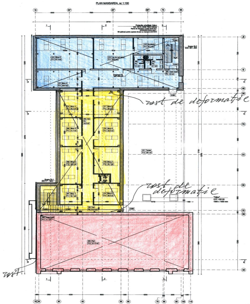
fig. 13. Plan mansarda. schema dispazitiei la blocuri seismice cu rosturi de deformatie
