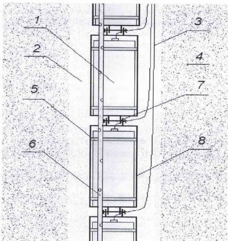
рис. 2 Анодный заземлитель комплектный глубинный – АЗК (Г).
