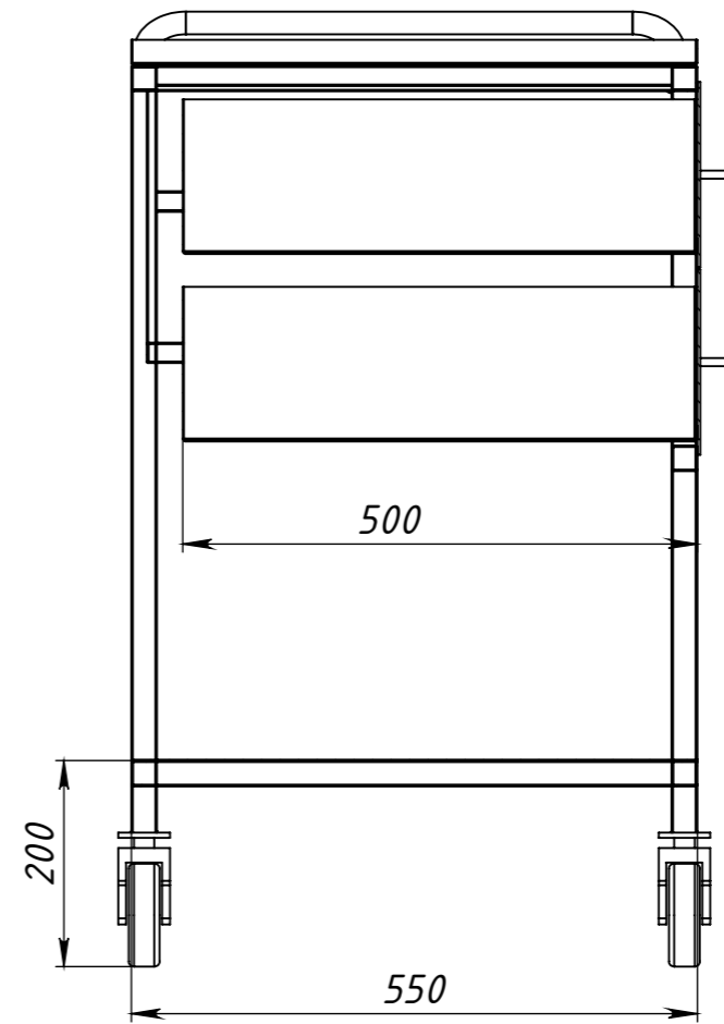
B-B (1 : 8)
