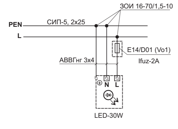
Schema de conectare a corpurilor de iluminat
