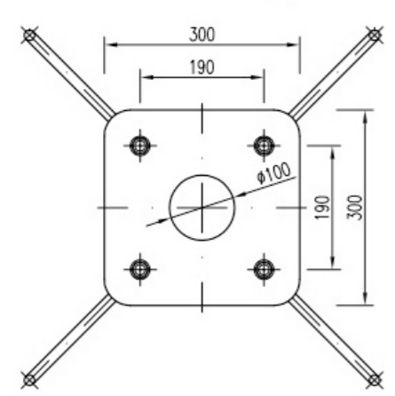
Арматура фундамета M16/190
