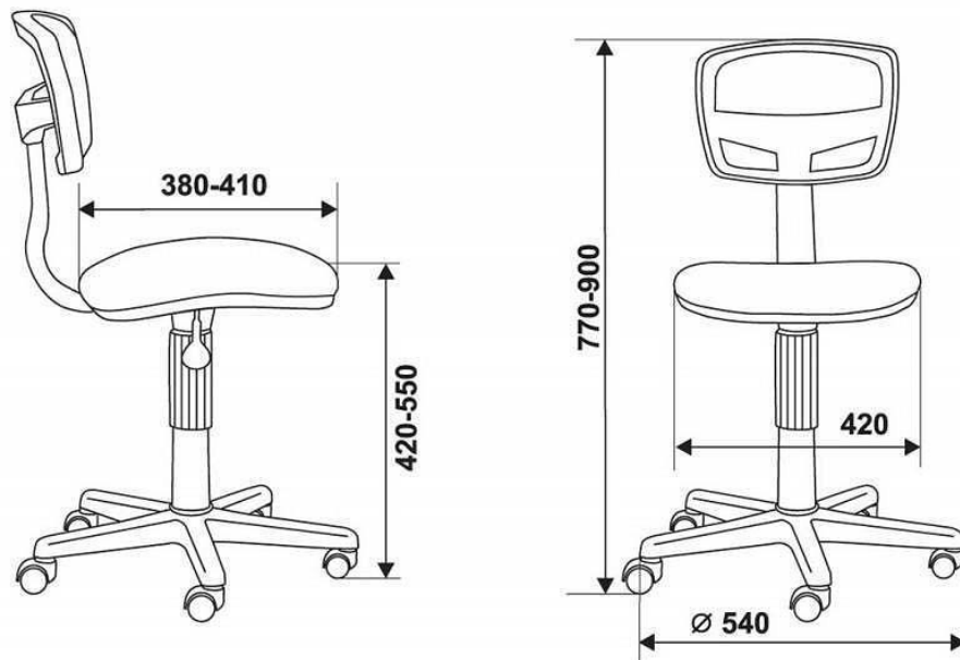
Desen 2. Scaun pentru laborator
