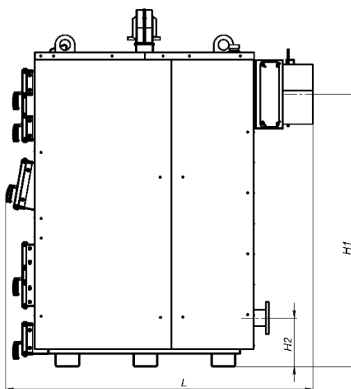
Рисунок 1 – Позначення габаритів котла
