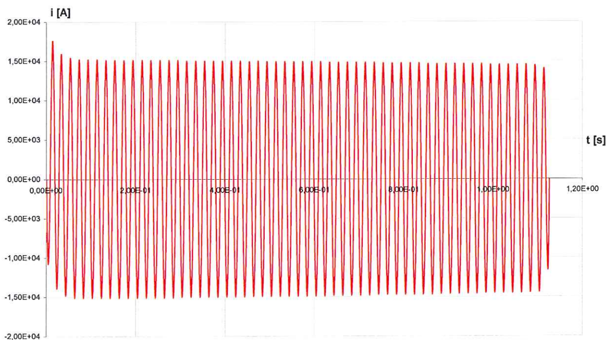
Oscylogram nr 1. Oscylogramy prądu zwarciovego
