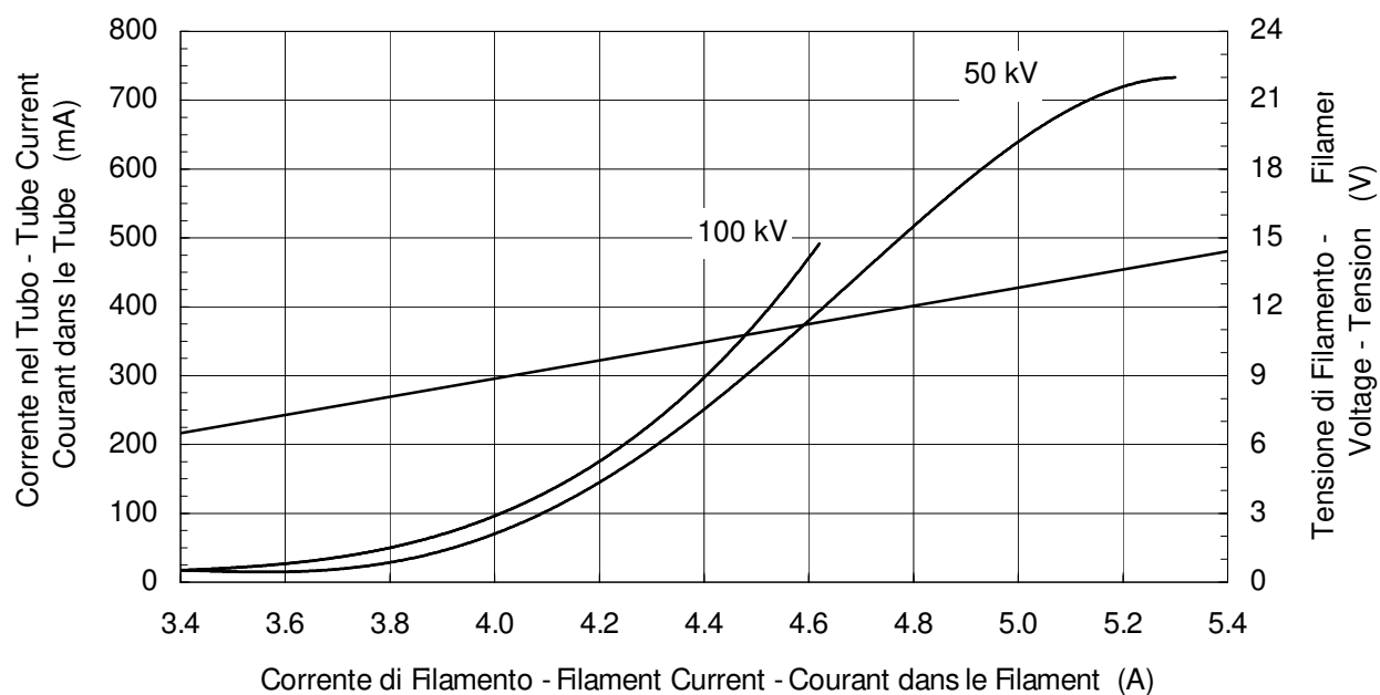
Caratteristica di emissione del catodo Cathode emission characteristic Caractéristique d'émission de la cathode ■ 1.2 - 3 ~ - ( \pm 0.2 A)
