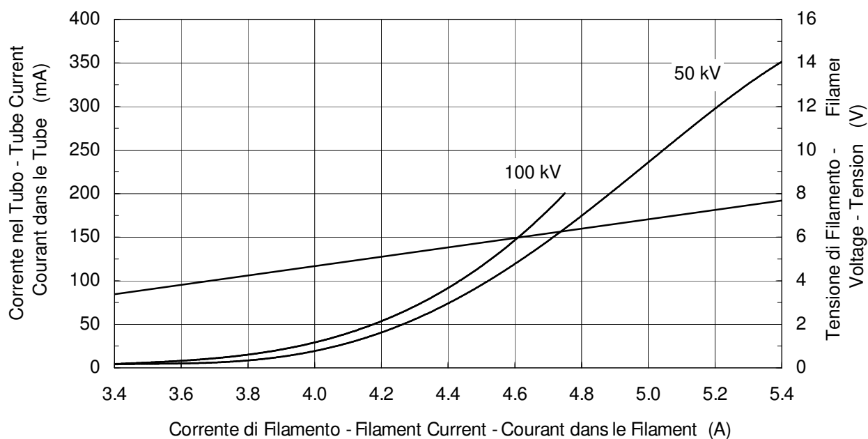
Caratteristica di emissione del catodo Cathode emission characteristic Caractéristique d'émission de la cathode ■ 0.6 - 3 ~ - ( \pm 0.2 A)
