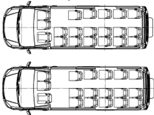
планировки салона
