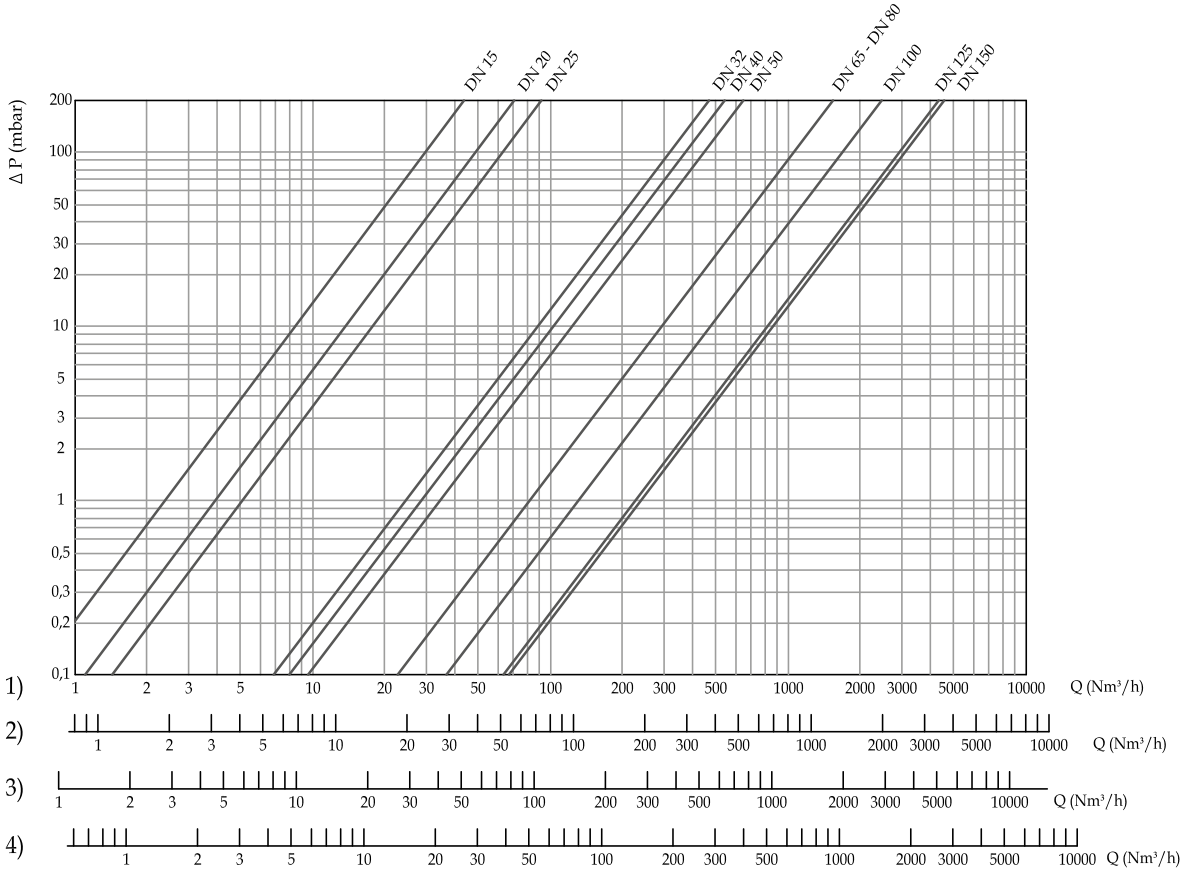
Диаграмма пропускной способности регулятора RG/2MC (без фильтра)
