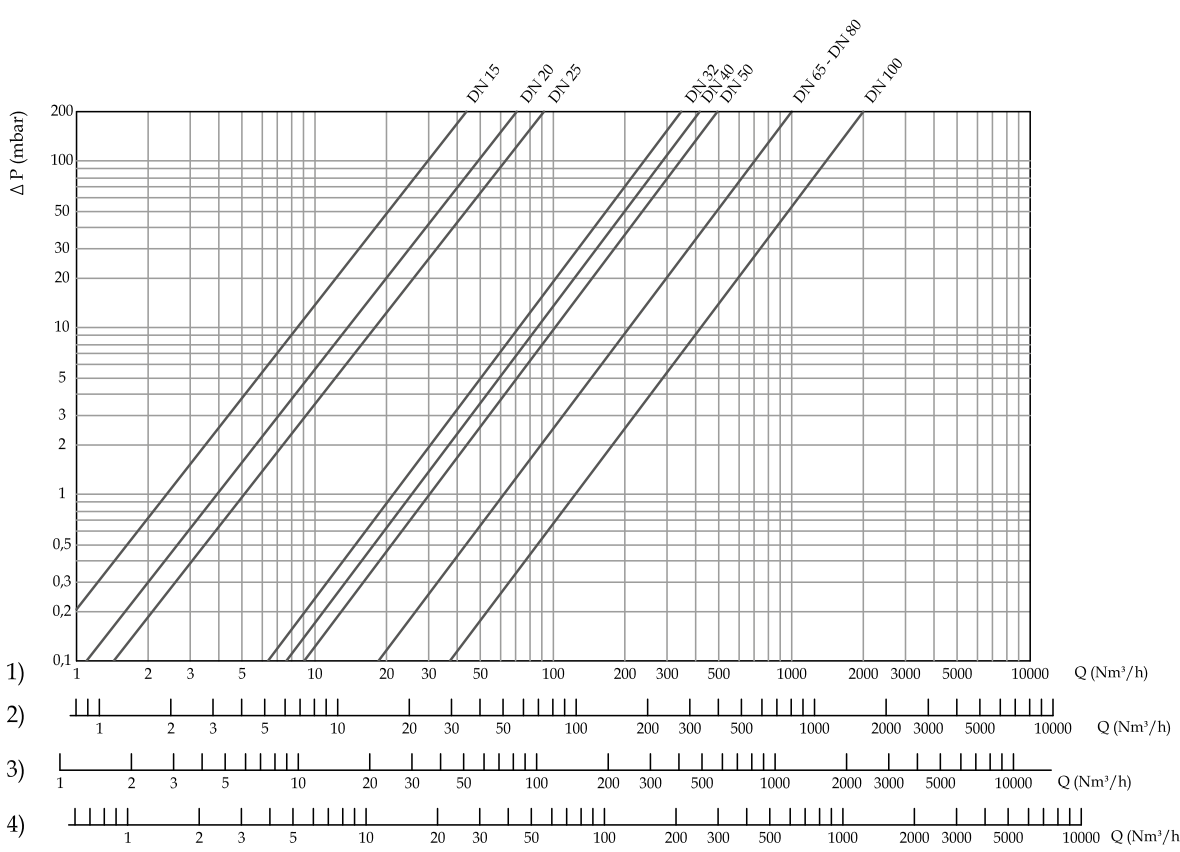
Диаграмма пропускной способности регулятора FRG/2MC (с фильтром)
