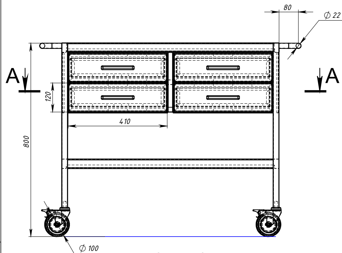
A-A (1 : 9)
