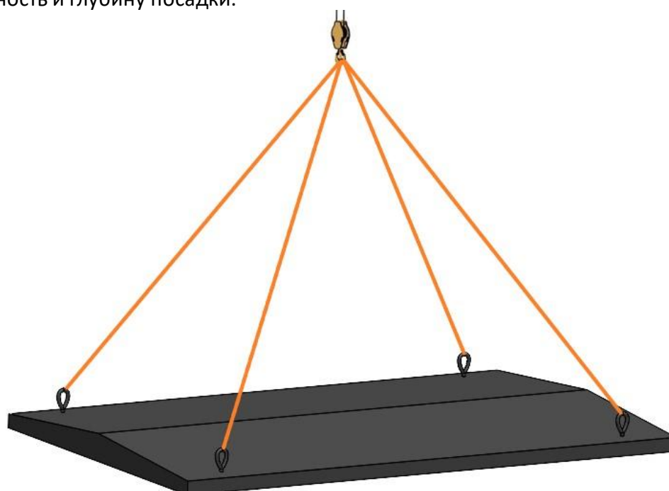
Рис. 4 Схема строповки крыши GALBOX.
