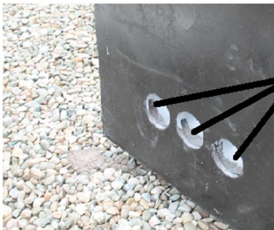
Рис.15 Отверстия для захода кабеля в фундамент GALBOX
