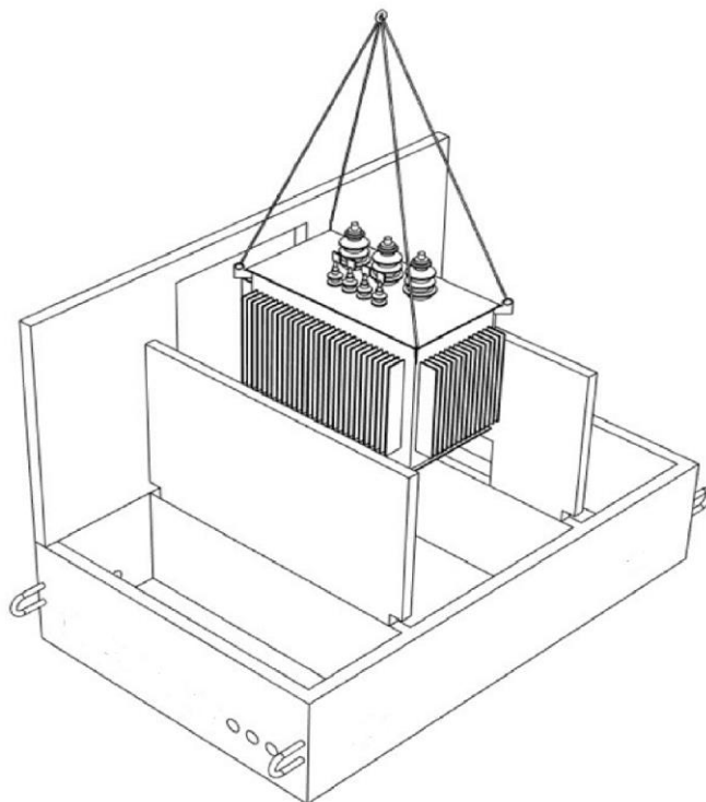
Рис.7 Монтаж трансформатора в корпус Galbox.
