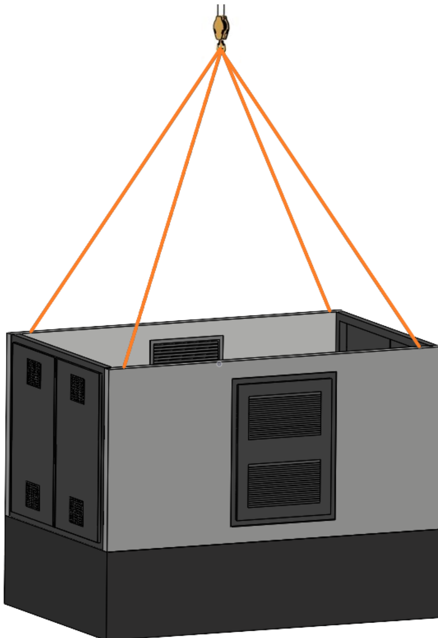
Рис.5 Пример разгрузки корпуса GALBOX.
