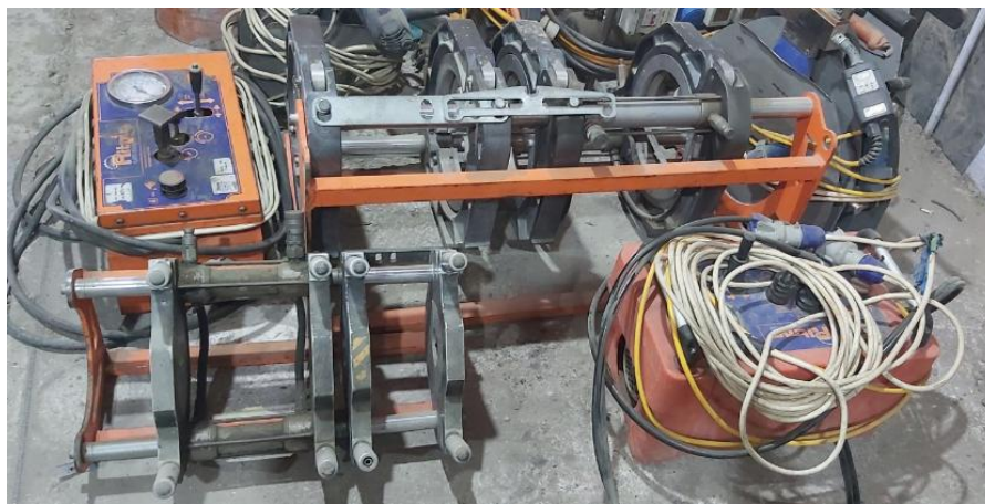
Figura 87. Vedere Nr.1
