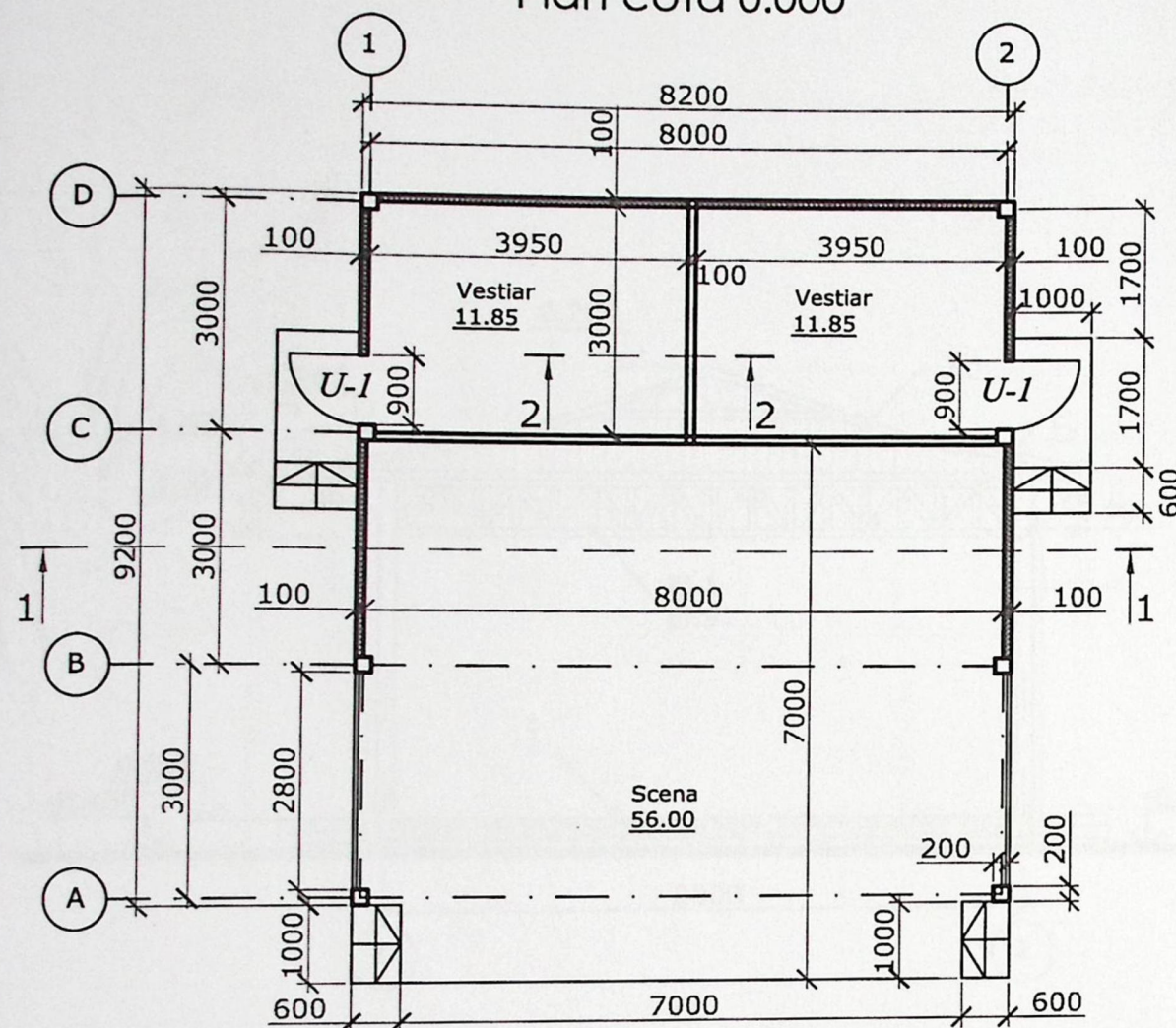
Plan cota 0.000
