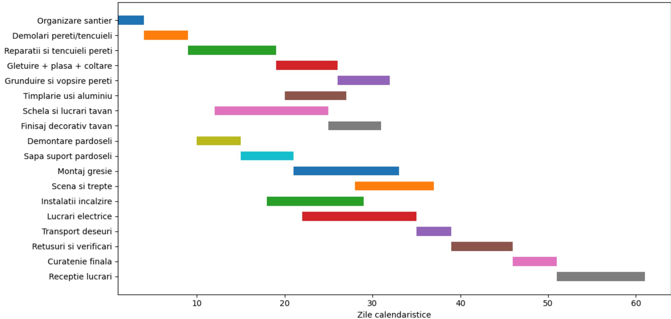
Grafic Gantt - Executarea lucrarilor (60 zile)
